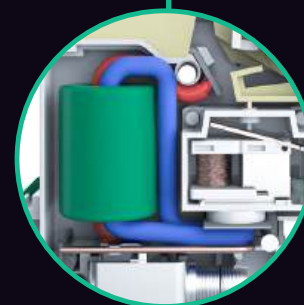
Электромеханический принцип действия
